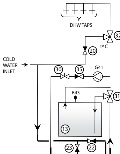
Bild 2. Extern varmvattentank
